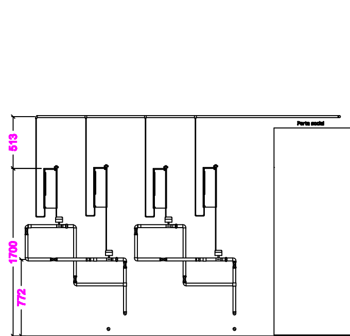
Corte CC
